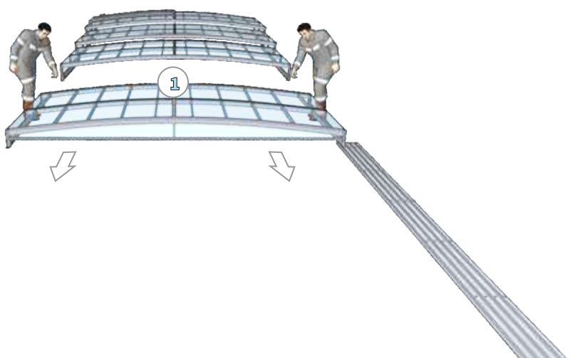
SEGMENT NR.1 / STEP - 2
